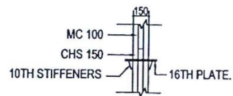
DETAIL-B
